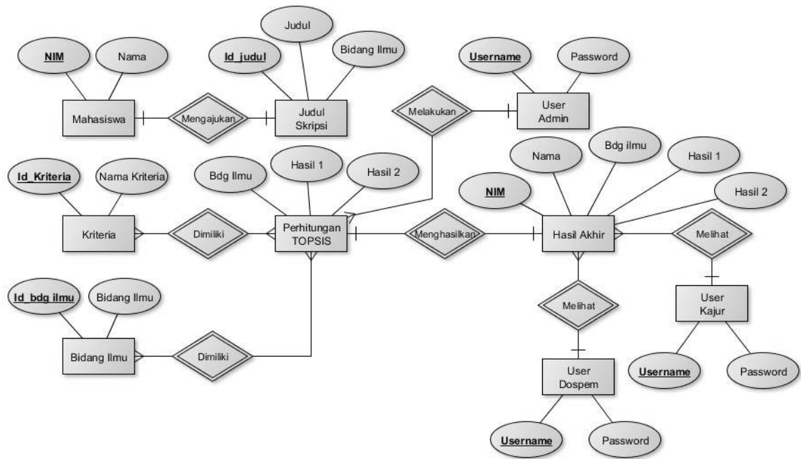
Gambar 3 ERD
