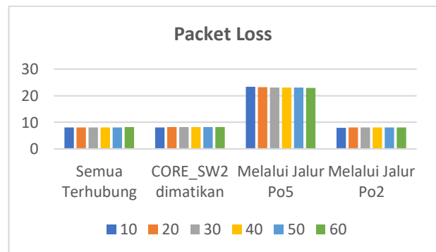
Gambar 5. Pengukuran Packet Loss disemua kondisi
